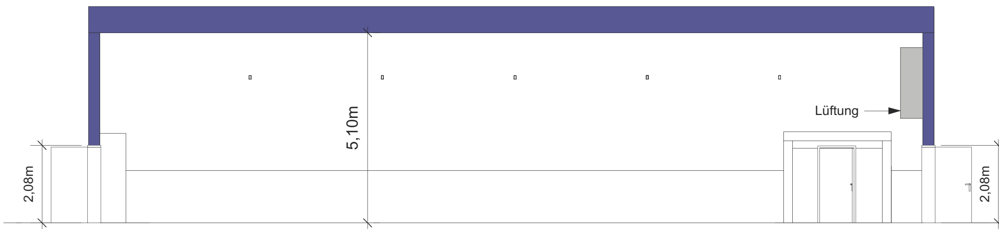
1 Längsschnitt 01 Maßstab: 1:100
