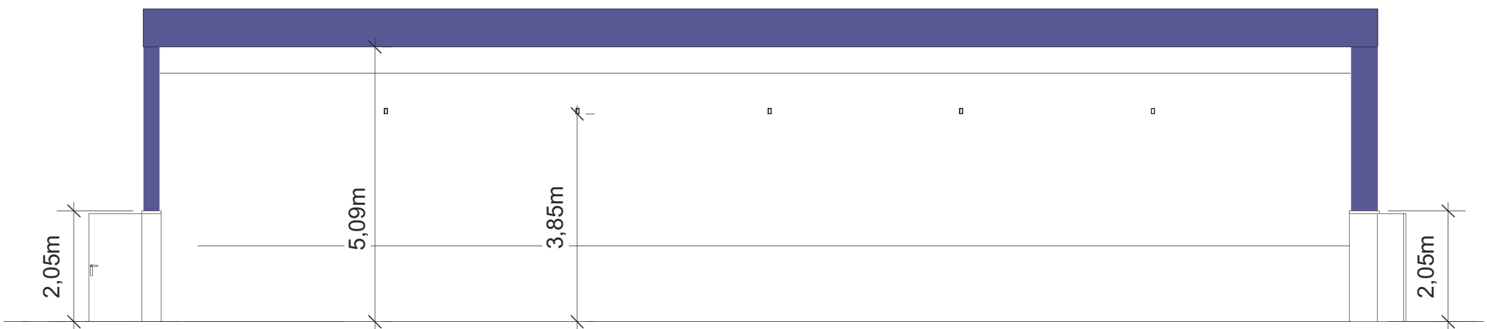
1 Längsschnitt 01 Maßstab: 1:100
