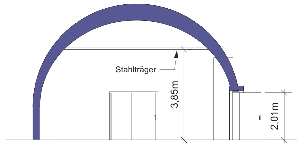
2 Querschnitt 01 Maßstab: 1:100
